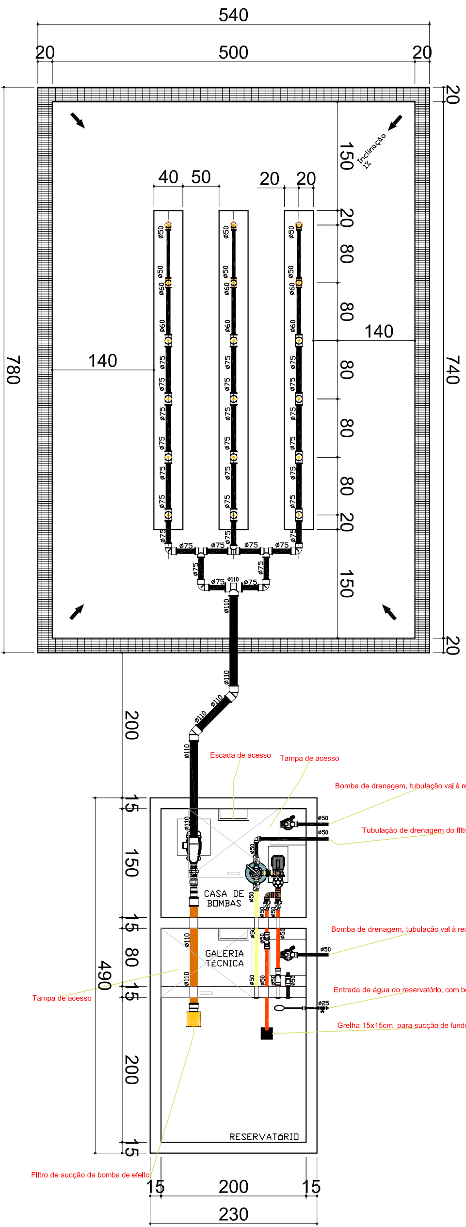
Planta hidráulica Escala: 1:150
