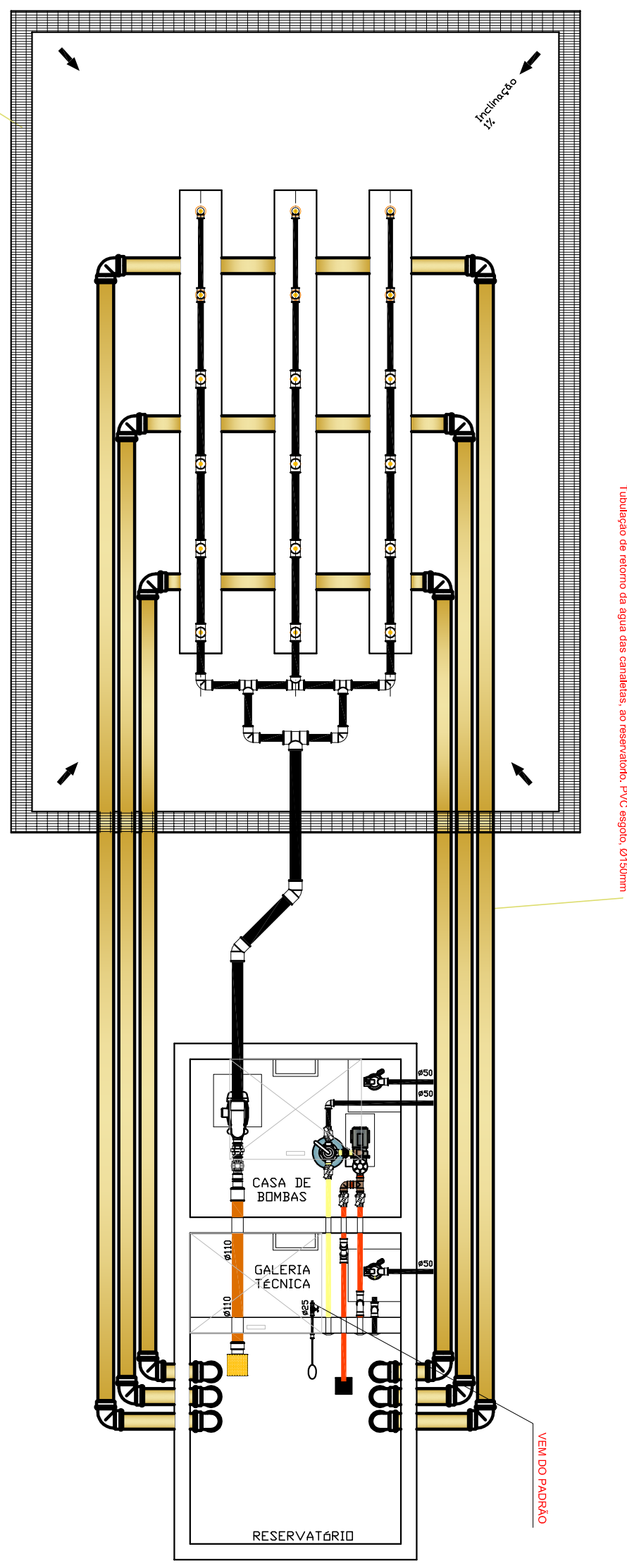
Planta hidráulica retorno Escala: 1:150
