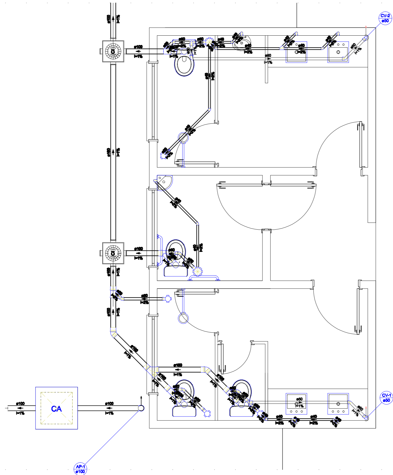
Térreo - Sanitário DETALHE SAN 2 1:25
